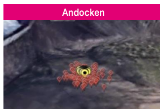
Vergleich der Standard-GNSS- und Precise-Positioning-Lösung in Pfadverfolgungs- und Andocktest Rote Punkte – Positionsbestimmung mit Standard-GNSS Gelbe Punkte – Precise Positioning
